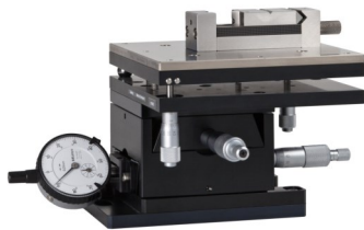
Modular aufgebauter Kreuztisch von LNP
